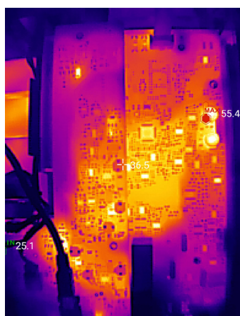
电路板
