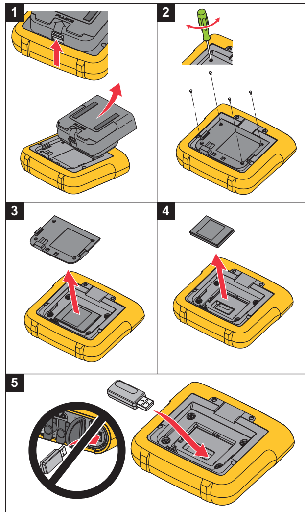
图示 1. 安装适配器
