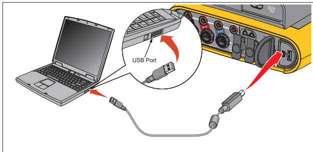
图示 8. Power Logger 至 PC 的连接
