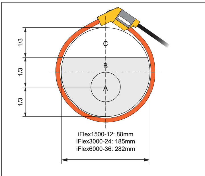
图示 9. iFlex 探头窗口
