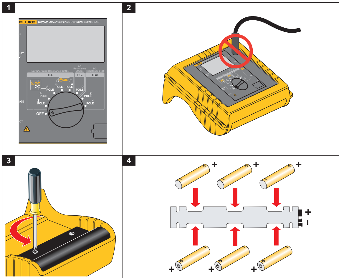
图 2. 电池插入
