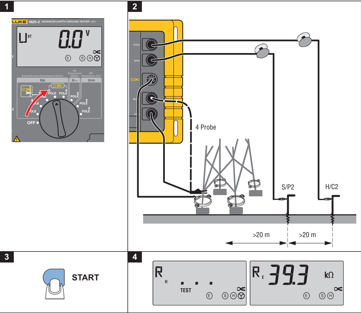
图 7. 不切断架空地线的接地电阻
